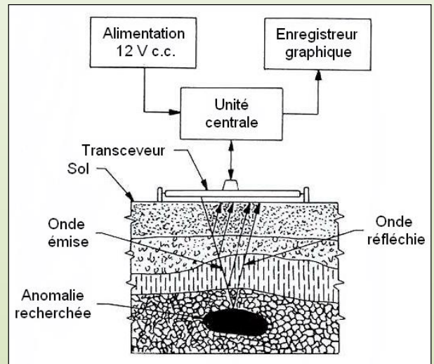
Principe de fonctionnement du géoradar
