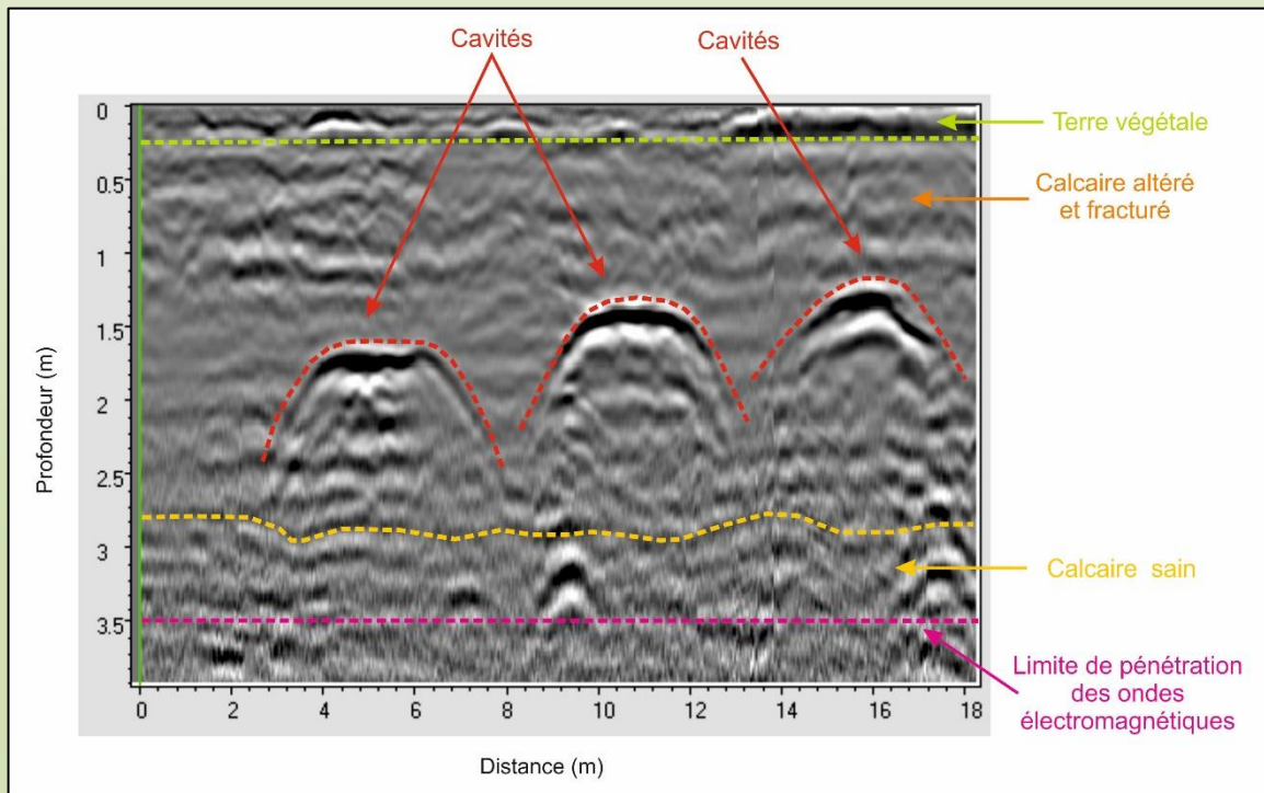
Radargramme commenté montrant la position de cavités karstiques
